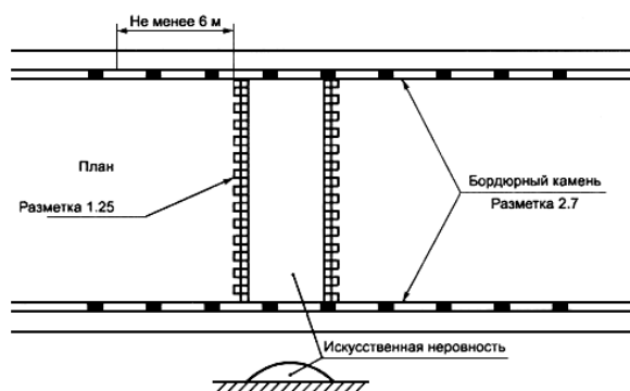
б - сборно-разборная конструкция
